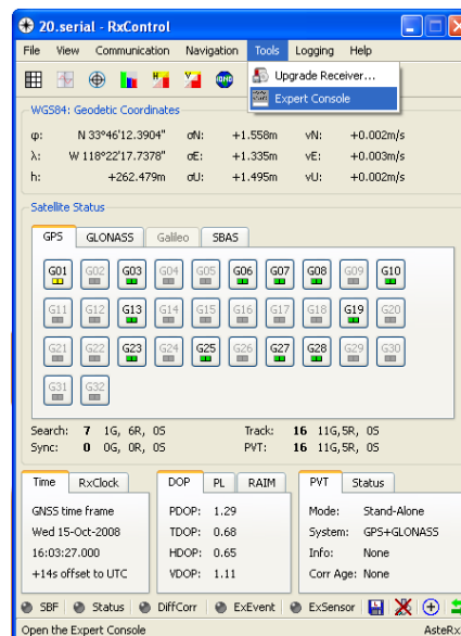
Рисунок 14: Экран RxControl
