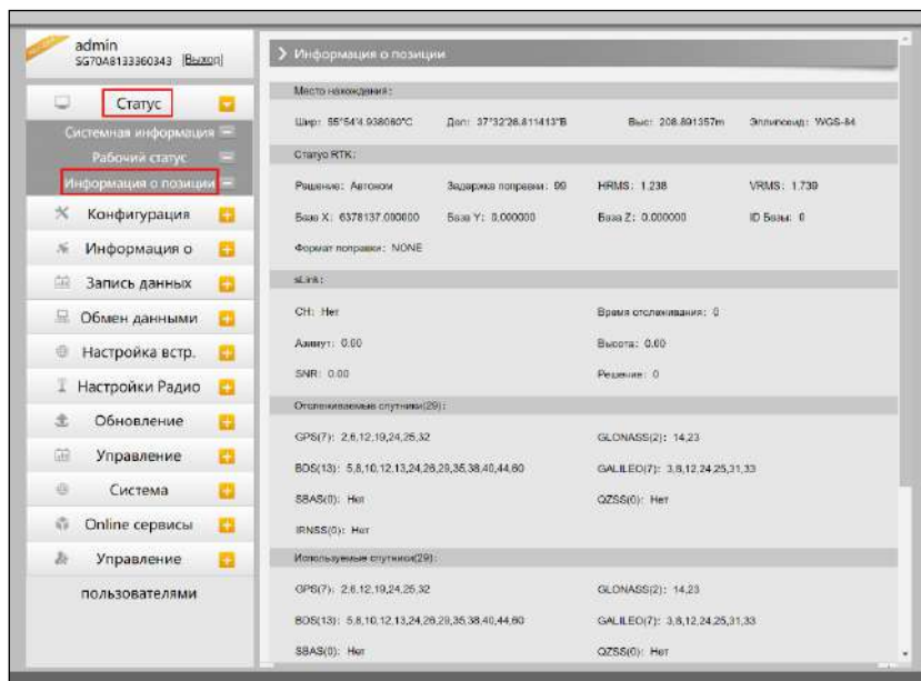
Изображение 2.4.3-3 Веб-интерфейс, вкладка Статус-Системная информация
