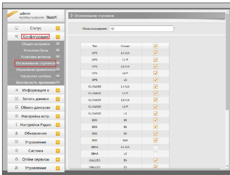
Изображение 2.4.4-4 Веб-интерфейс, вкладка Конфигурация-Отслеживание спутников
