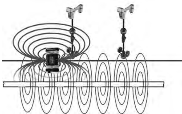
Рис. 12: Вблизи передатчика приемник принимает местное поле диполя, созданное вокруг передатчика.
