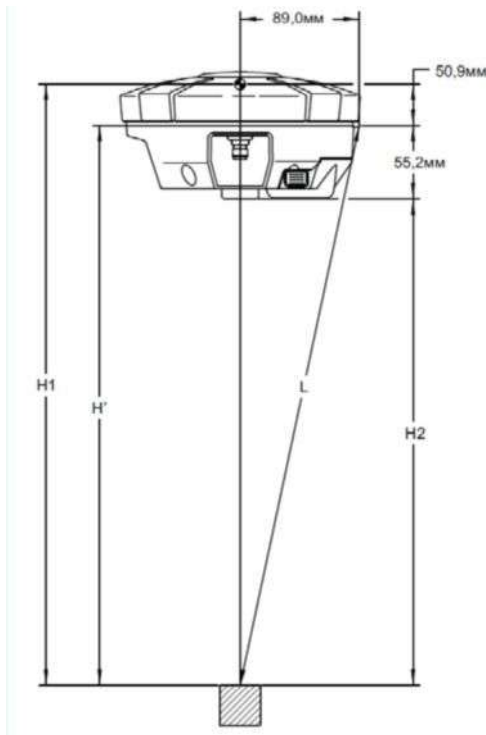
Рис. 4-3. Измерение высоты антенны
