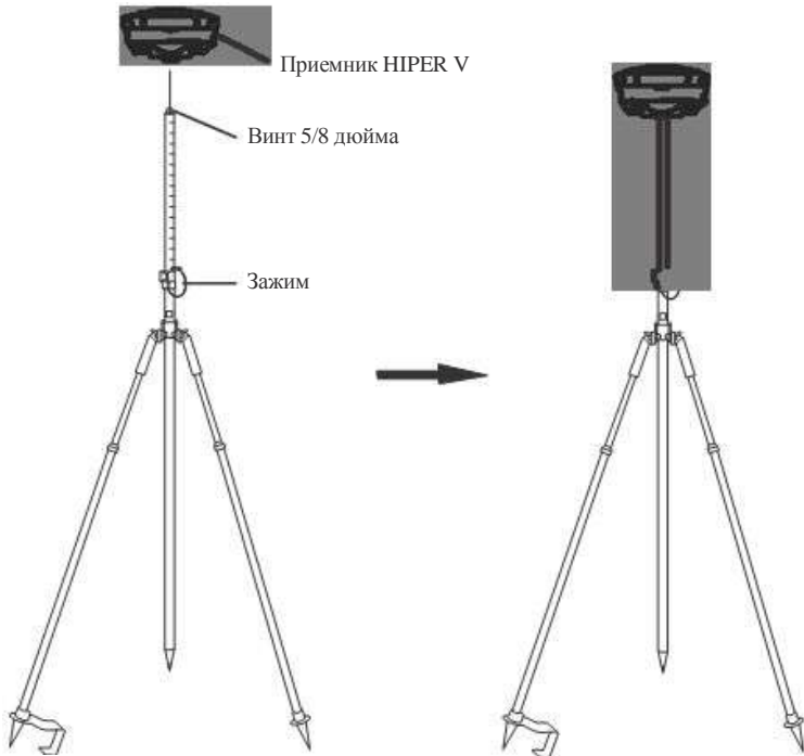
Рис. 4-2. Крепление HIPER V на вешке к биподу
