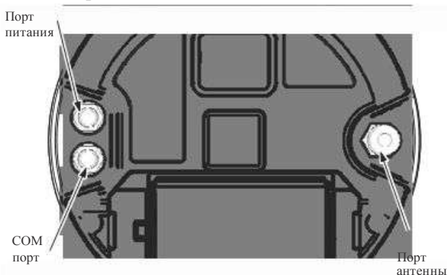
Рис. 1-4. Порты приемника HIPER V
