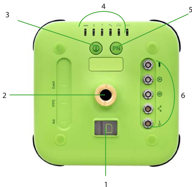
Рисунок 2. ТРИУМФ-1М
