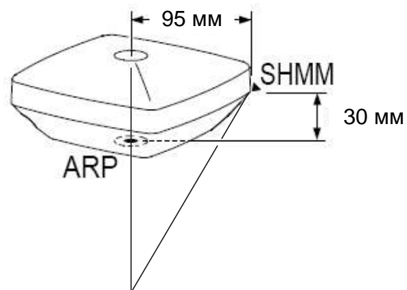
Рис. 18: Точки измерения высоты антенны
