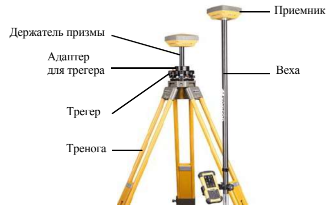
Рис. 15: Оборудование и конфигурация
