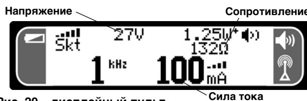
Рис. 20 – дисплейный пульт
