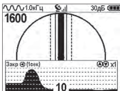
Рис.А.3 КЗ-однофазное
