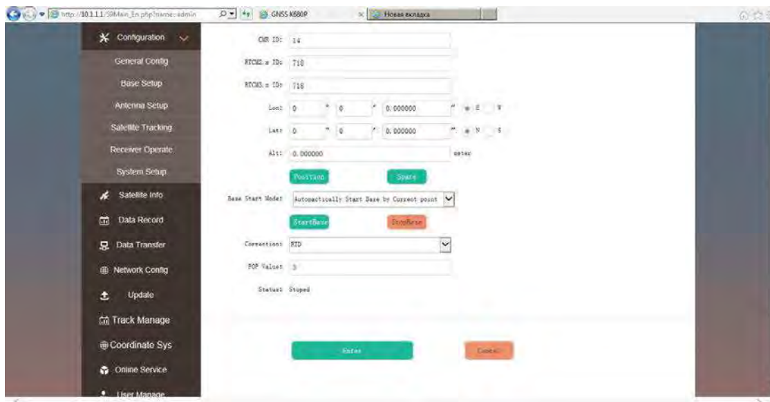
Рисунок 2.3.9 Настройка базы
