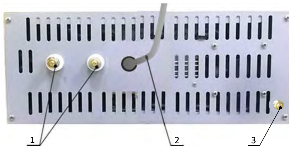
Рисунок 2. Задняя стенка генератора.
