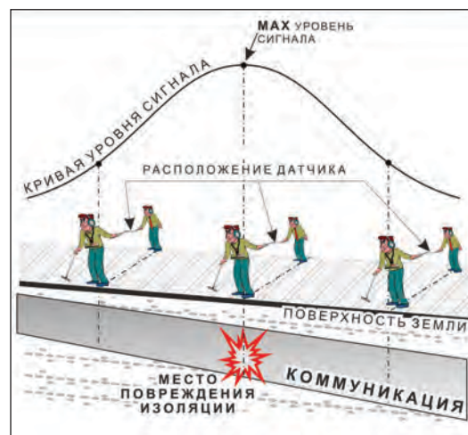
применение датчика-определителя дефектов коммуникации (ДОДК) методом max
