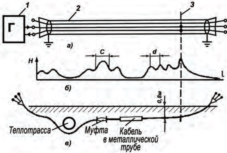
Рис.5.11 КЗ-междуфазное
